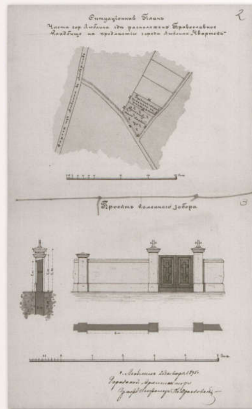
Plan sytuacyjny i projekt ogrodzenia ementarza prawosławnego, dawnego unickiego, na Czwartku (róg ulic Unickiej i Walecznych), 1895 r.
