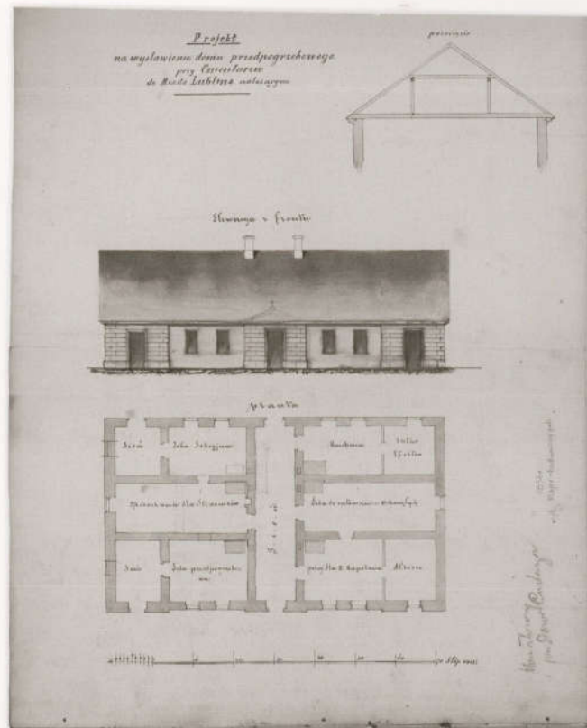
Projekt domu pogrzebowego na cmentarzu miejskim przy ul. Lipowej, 1854 r.
