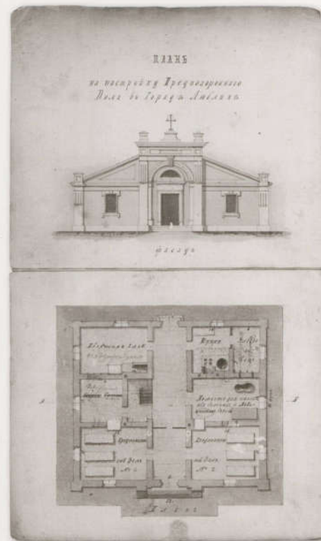
Projekt domu pogrzebowego na cmentarzu miejskim przy ul. Lipowej, 1871 r.
